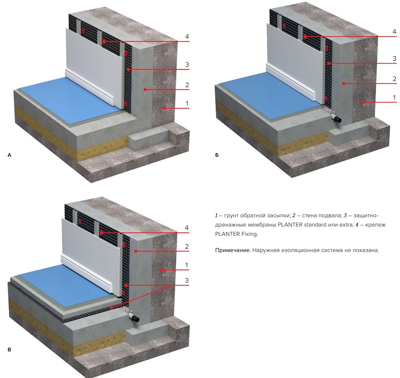
Конструктивные схемы изоляционных систем при ремонте влажных стен подвала
